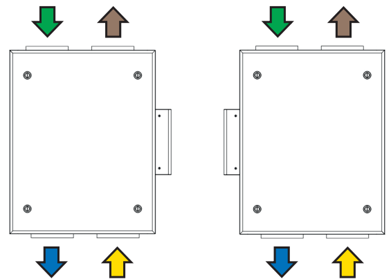
CASA R9-H L, vänsterutförande
