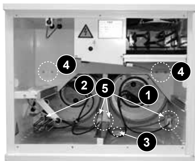
1. Poistoilmapuhallin 2. Tuloilmapuhallin 3. Kondenssiveden poistoviemäri 4. Puhaltimien lukitsinsalvat 5. Puhaltimien pistokeliitännät
