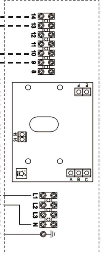
Elvärmarens anslutningslåda
