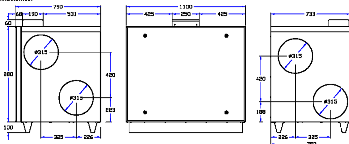
Måttskiss:
